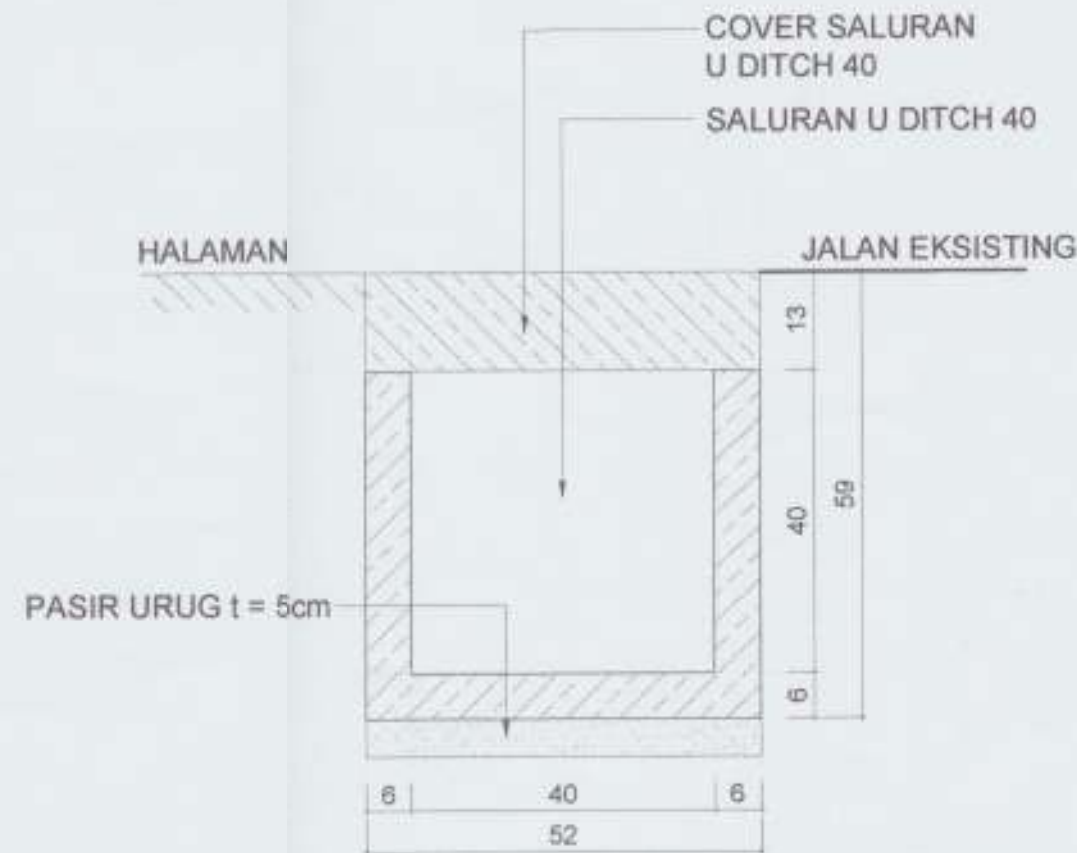
DETAIL SALURAN U DITCH 40 Skala 1 : 10
