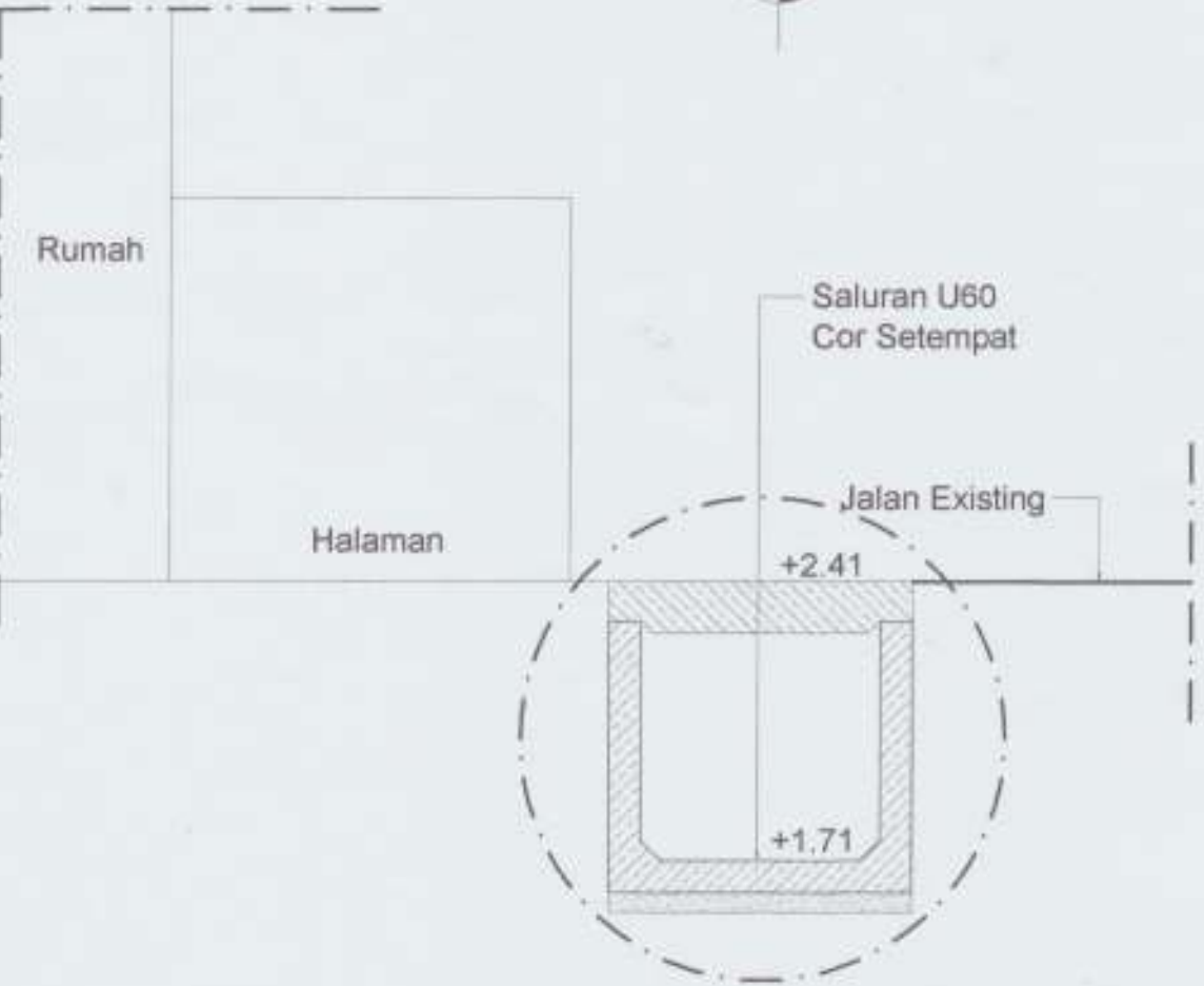
POTONGAN A RENCANA S5 Skala 1 : 20
