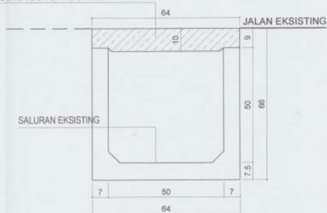
DETAIL SALURAN U DITCH 50 Skala 1 : 10
