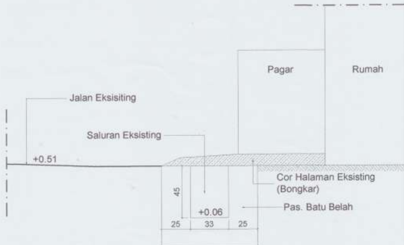
POTONGAN A EKSISTING S1A Skala 1 : 20
