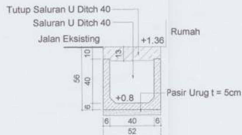
DETAIL SALURAN U DITCH 40 Skala 1 : 20
