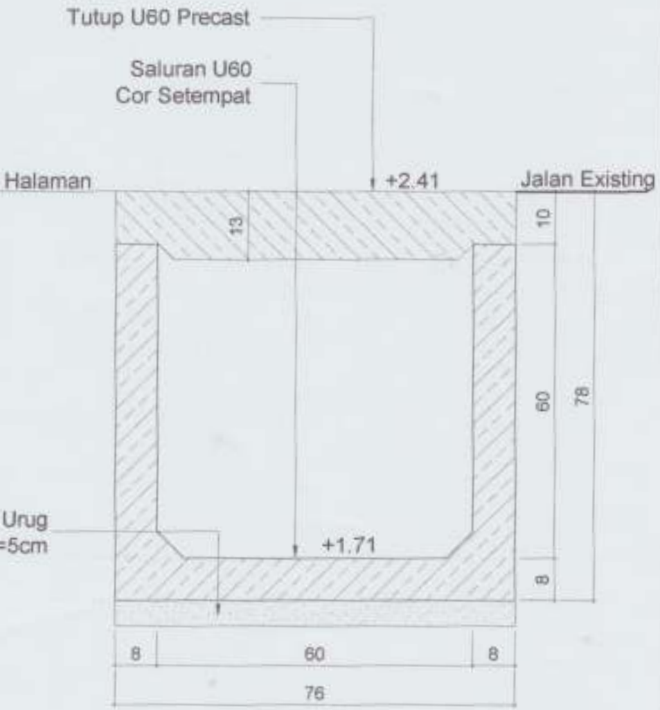
DETAIL SALURAN U60 COR SETEMPAT Skala 1 : 10
