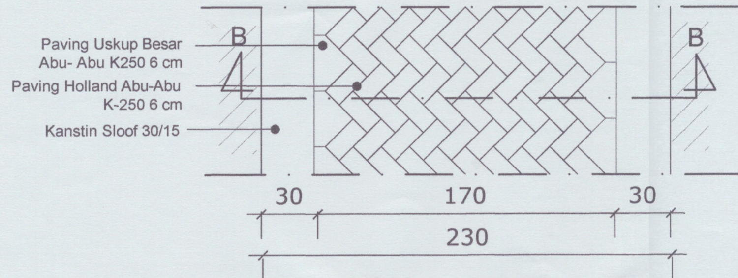
T. ATAS JP3 RENCANA Skala 1:20
