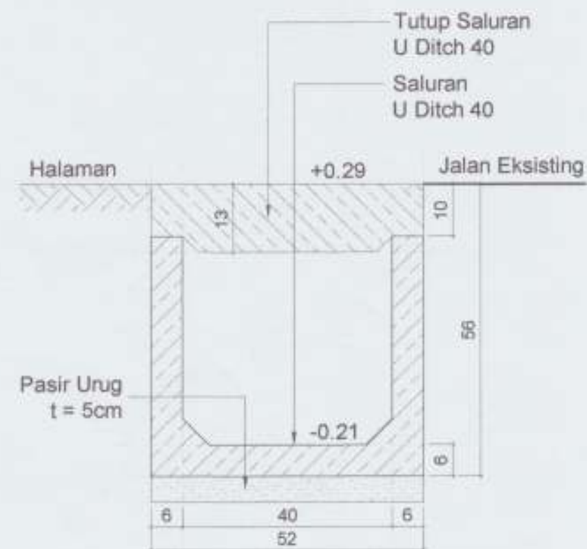
DETAIL SALURAN U DITCH 40 Skala 1 : 10
