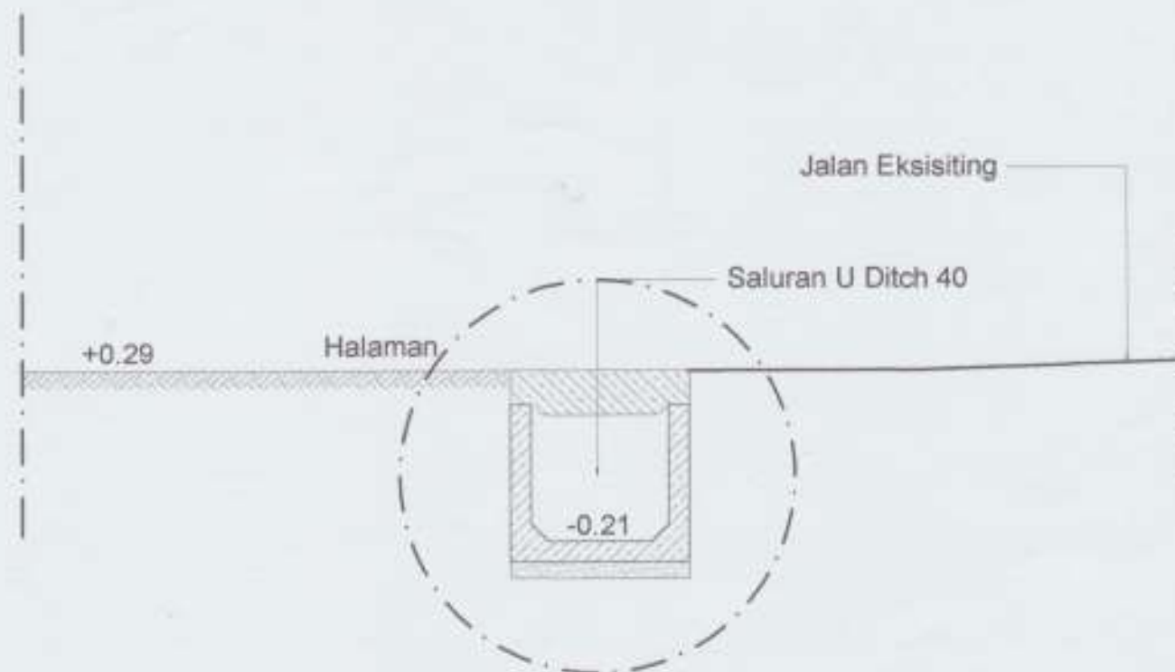
POTONGAN B RENCANA S1A Skala 1 : 20
