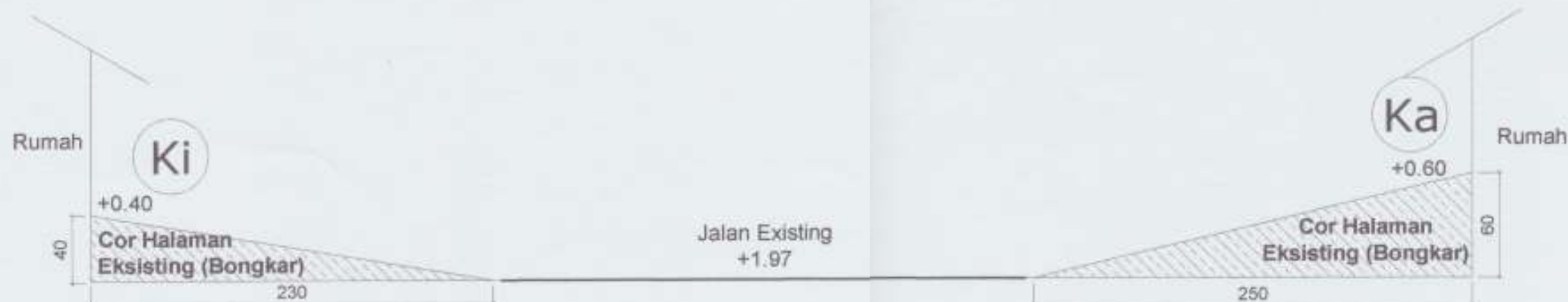
POTONGAN B EKS. S3 Skala 1 : 40
