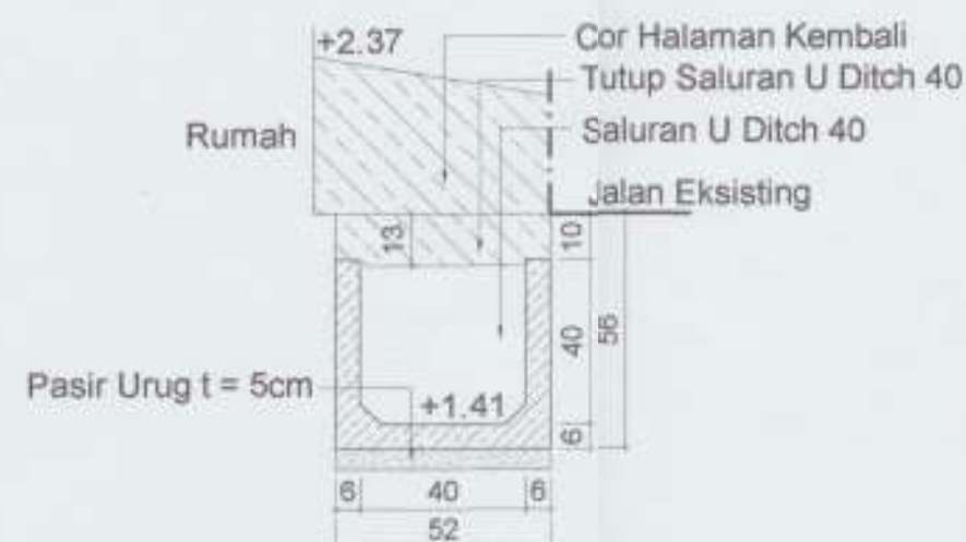
DETAIL SALURAN U DITCH 40 Skala 1 : 20
