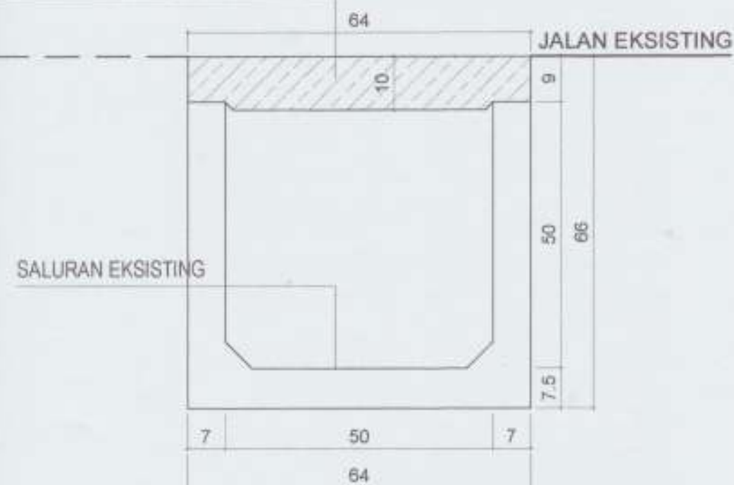
DETAIL SALURAN U DITCH 50 Skala 1 : 10
