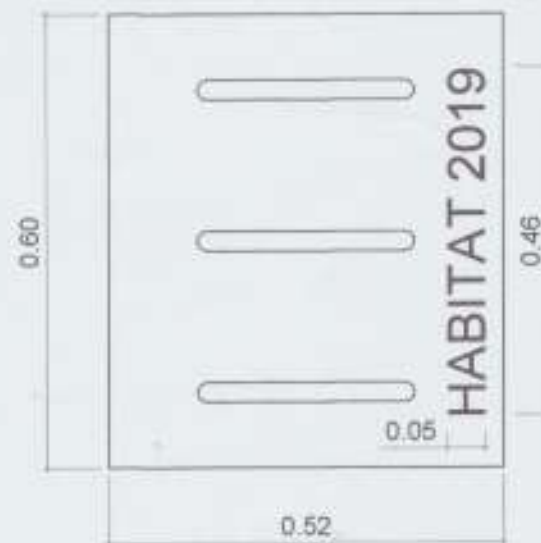
COVER SALURAN U DITCH 40 DENGAN TULISAN HABITAT 2019 Skala 1 : 10
