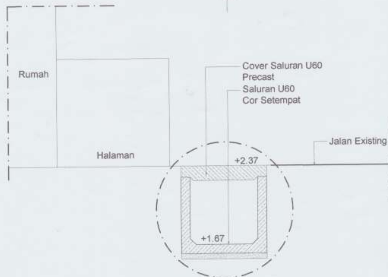
POTONGAN B EXISTING S5 Skala 1 : 20
