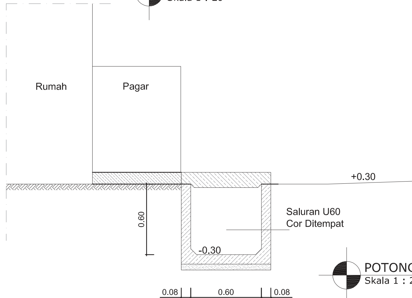
POTONGAN A EKSISITING S2 Skala 1 : 20
