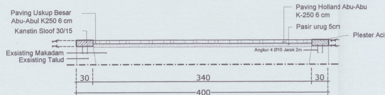
POTONGAN B-B Skala 1: 40
