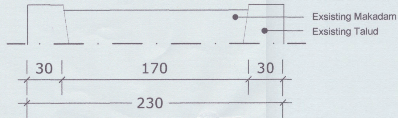
EXISTING JP3 Skala 1:20
