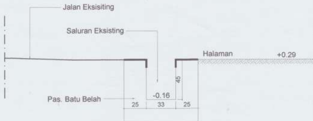
POTONGAN B EKSISITING S1A Skala 1 : 20
