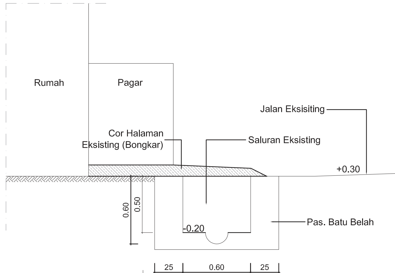
POTONGAN A EKSISITING S2 Skala 1 : 20
