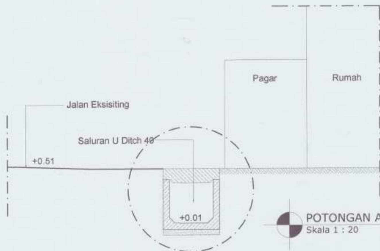
POTONGAN A EKSISTING S1A Skala 1 : 20
