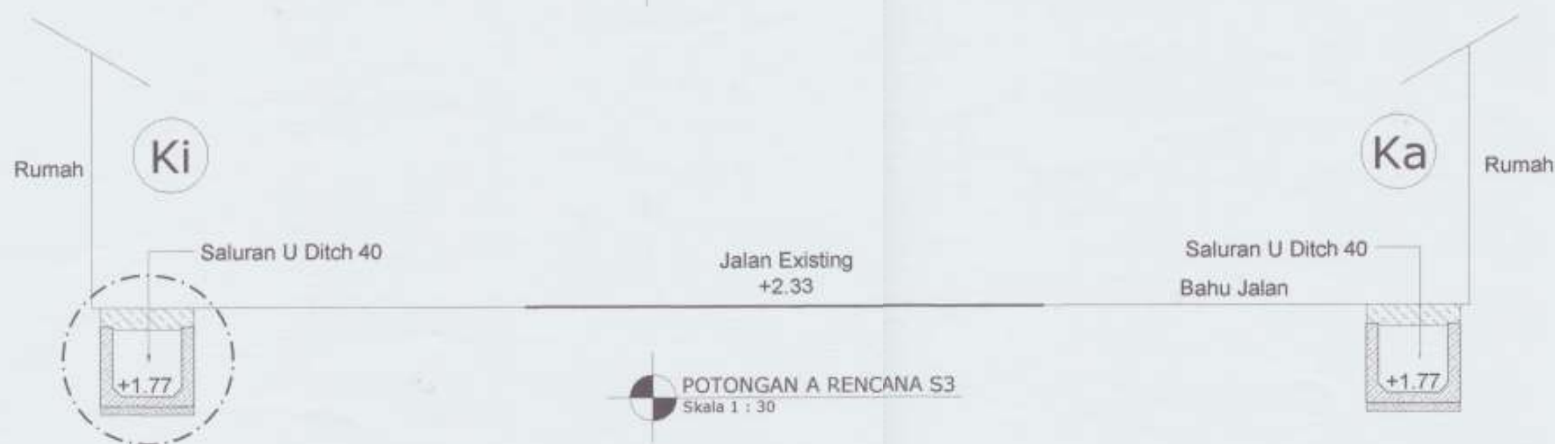
POTONGAN A EKSISTING S3 Skala 1 : 40
