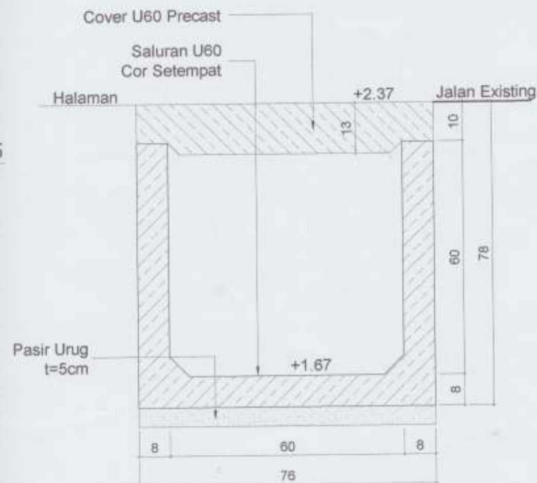
POTONGAN B EXISTING S5 Skala 1 : 20
