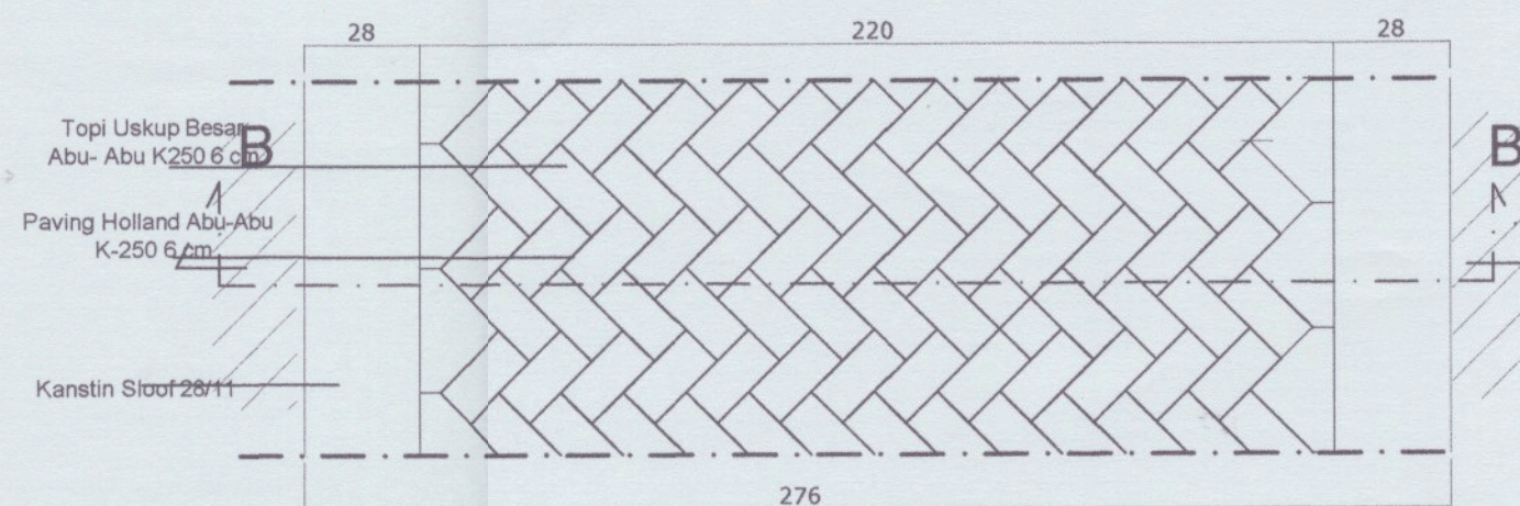
TAMPAK ATAS JP2 RENCANA Skala 1: 20
