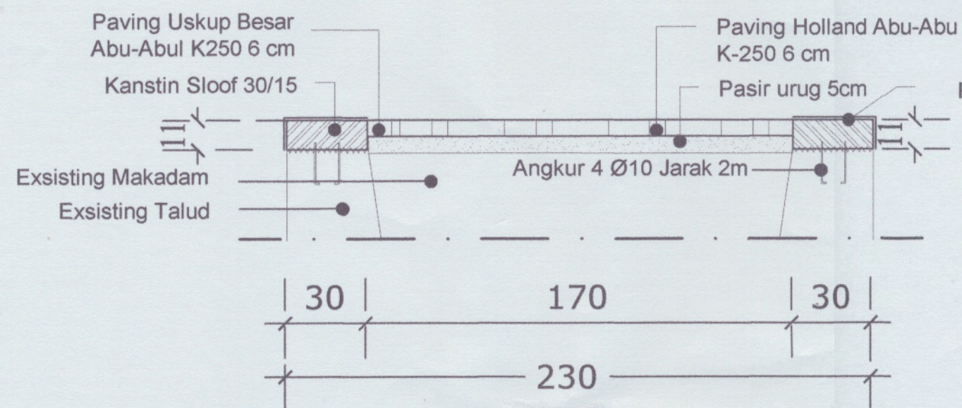
POTONGAN B-B Skala 1:20
