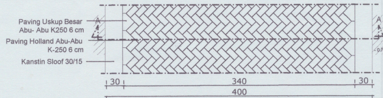
T. ATAS JP4 RENCANA Skala 1: 40
